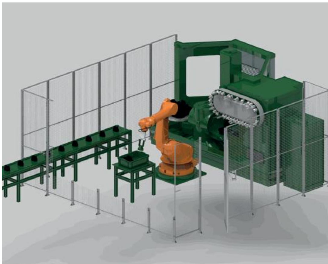
Рисунок А.1 – Пример контролируемой остановки с расчетной безопасностью
